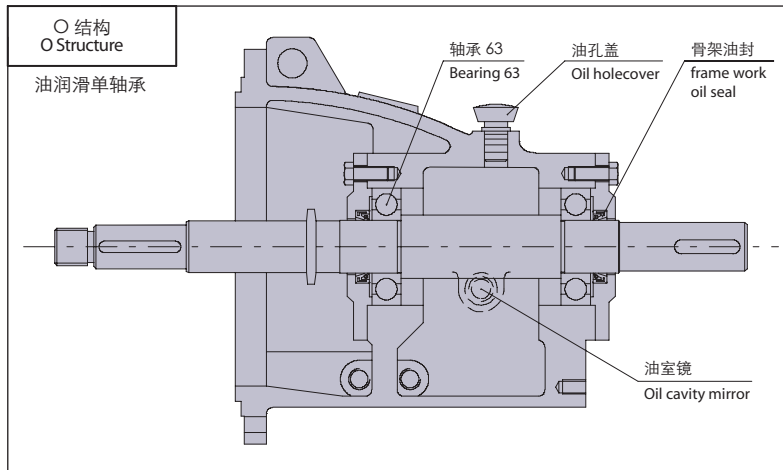
O结构：油润滑结构，适用所有泵型(可选配置)。 O structure: lubrication structure, suitable for all pump models(Optional).
