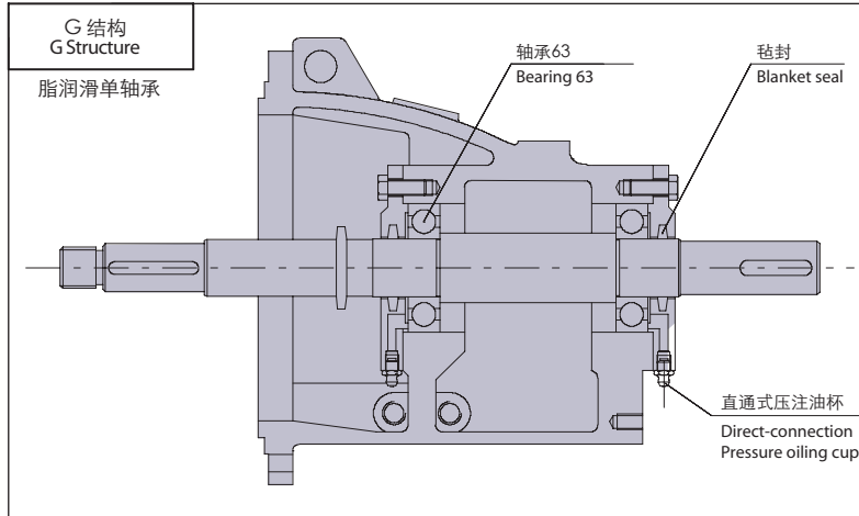
G结构：脂润滑结构，适用所有泵型(标准配置)。 G structure: grease lubrication structure, suitable for all pump models (Standard).
