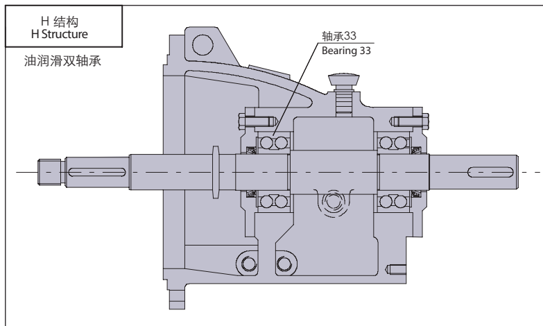
H结构：单指GHS 40/320；GHS50/320；GHS65/320；GHS80/320以上四型泵，可配置高速泵用。 H structure: only suitable for pump models of GHS40/320, GHS50/320, GHS65/320 and GHS80/320.
