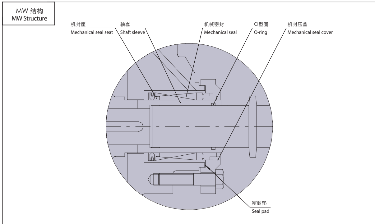
MW结构: 外装式非平衡式机械密封结构。 MW structure: outside-fitted non-equilibrium mechanical seal structure.
